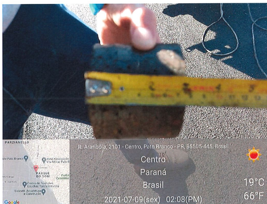
Foto 06: Extração corpo-de-prova Rua Urbano Wittmann
