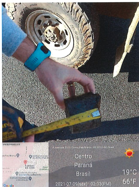
Foto 05: Extração corpo-de-prova Rua Urbano Wittmann
