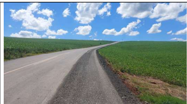
FOTO 04: BASE DE BRITA GRADUADA
