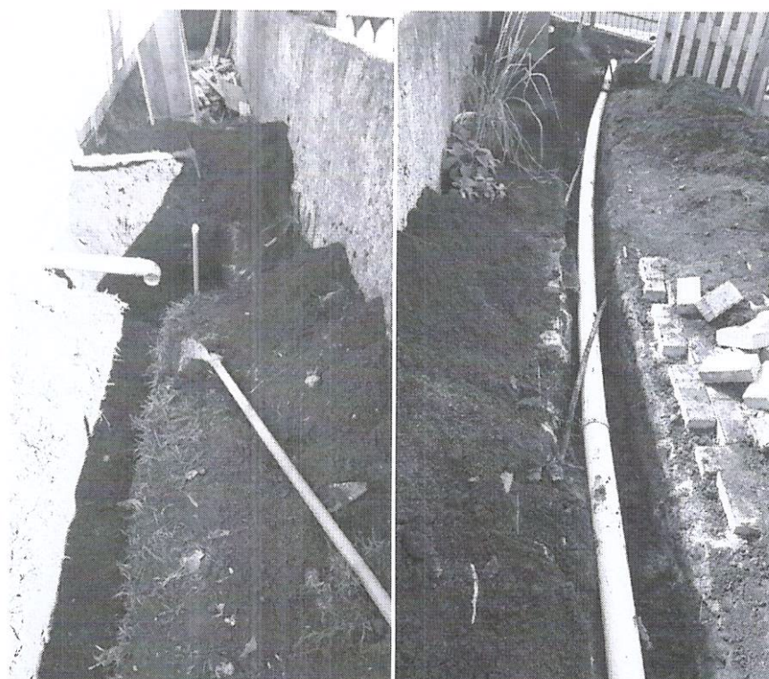
Foto 02: Instalação de tubulação sanitária
