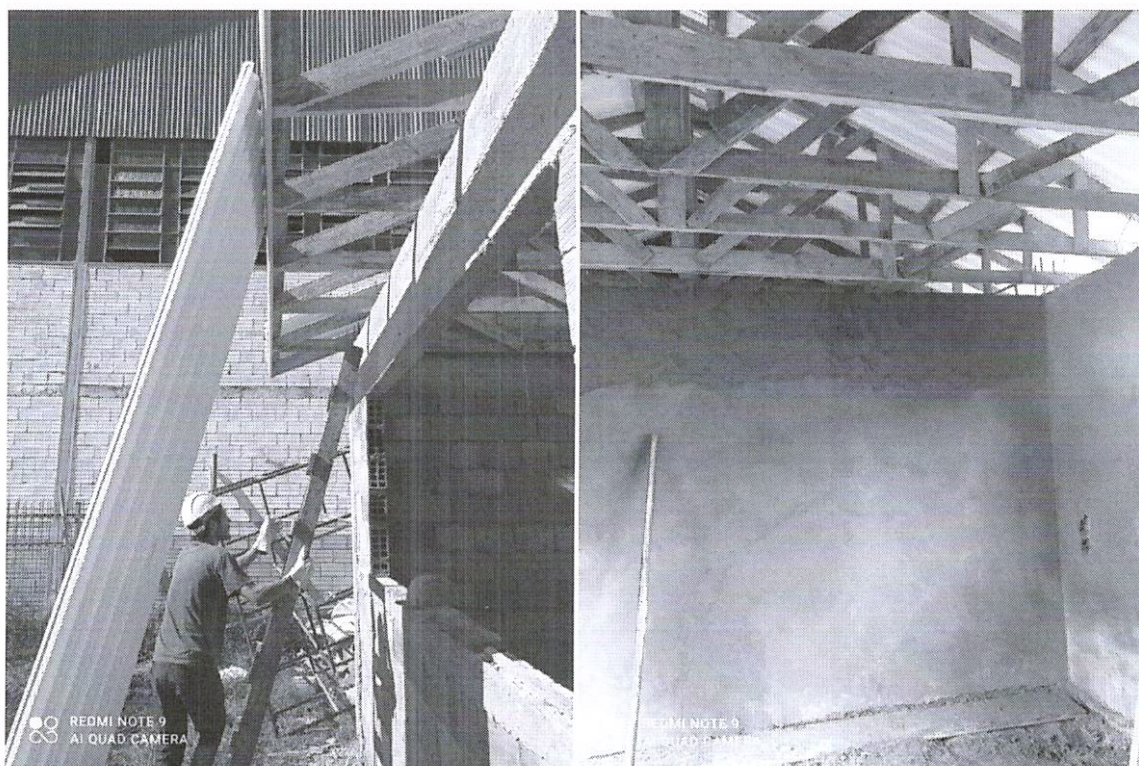
Foto 03: Estrutura Telhados
