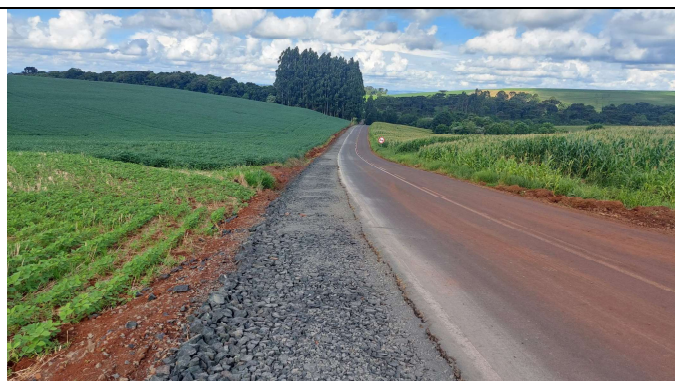
FOTO 07: SUB-BASE EM MACADAME
