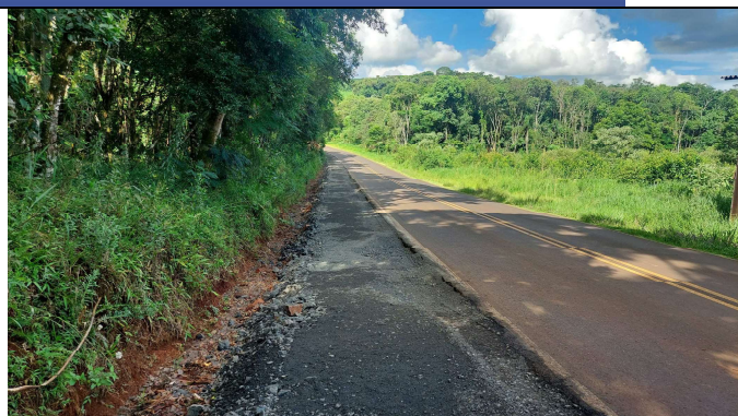
FOTO 05: SUB-BASE EM MACADAME
