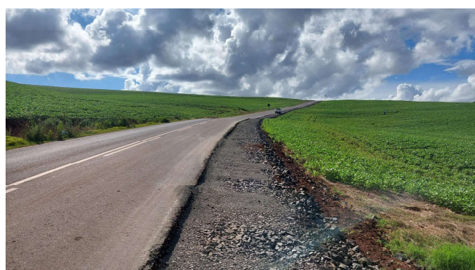
FOTO 08: SUB-BASE EM MACADAME
