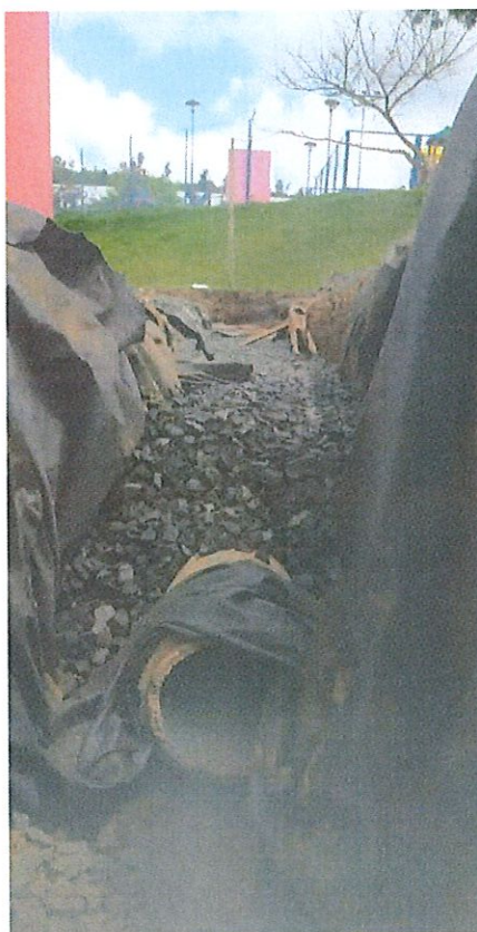
Foto 6: Trincheiras drenantes durante o processo de construção (obs: foram fechadas com camada de terra e aguardam a plantação das moreias para a próxima medição)
