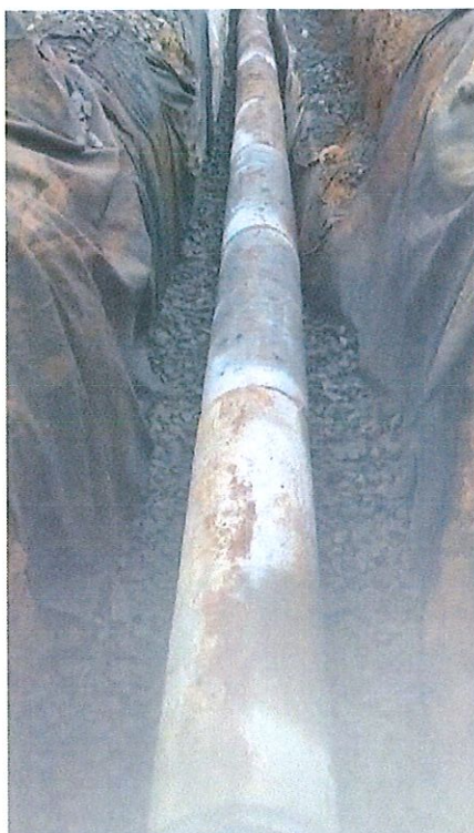
Foto 5: Trincheiras drenantes durante o processo de construção
