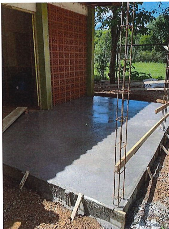
Foto 8: Radier concretado
