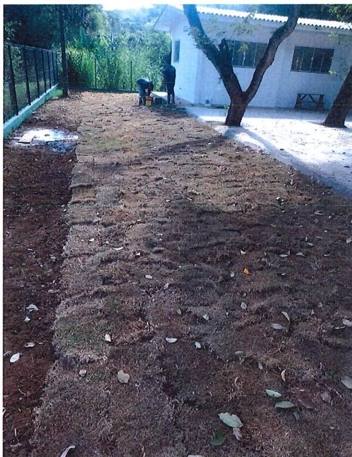
Foto 6: Execução de dreno / Plantio de Grama
