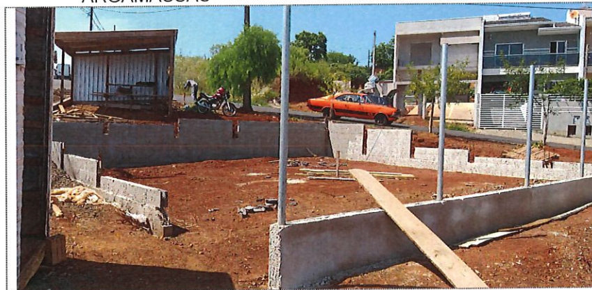
Impermeabilização de vigas baldrame no entorno do playground
