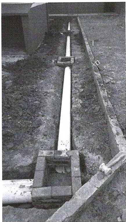
Foto 05: Tubulação assentada.
